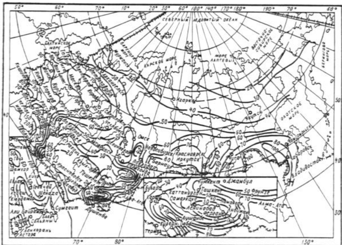
Черт. 1. Значения величин интенсивности дождя q_{20}
