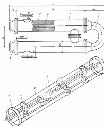
Рис. 2 Конструктивные размеры водоподогревателя
