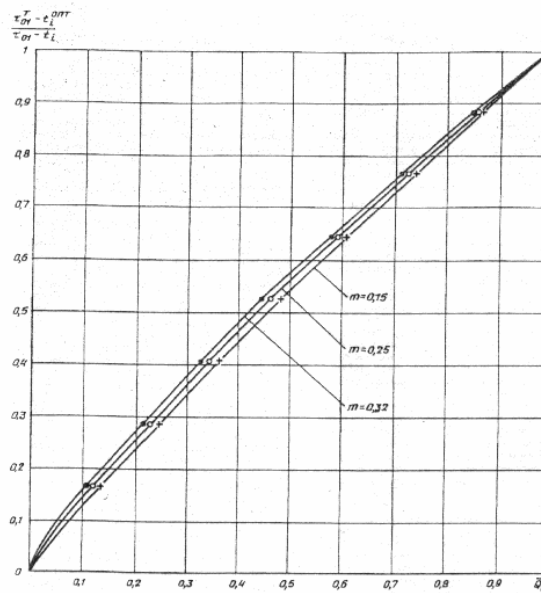
Рис. 2. Графики изменения температурного критерия системы отопления по температуре воды в подающем трубопроводе — \left( \frac{\tau_{01}^T - t_i^{\text{OPT}}}{\tau_{01}^T - t_i} \right) для различных значений показателя степени m и при постоянной циркуляции теплоносителя в системе
