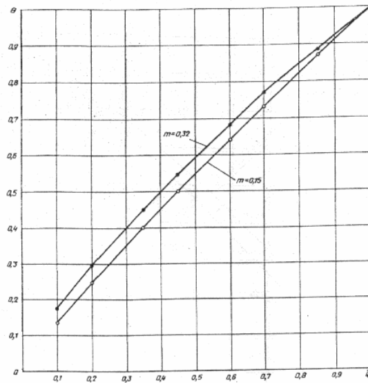
Рис. 4. Графики изменения относительных температур теплоносителя в одноконтурных системах отопления при количественно-качественном регулировании
