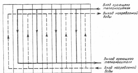
Рис. 1. Симметричная компоновка пластинчатого водоподогревателя, обозначение Сх 4/5
