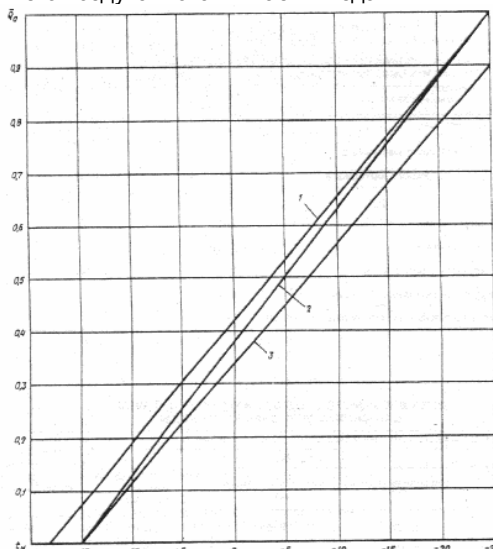
Рис. 1. Графики относительного изменения теплового потока на отопление Q_0 , в зависимости от наружной температуры t_0 для разного типа потребителей и способов авторегулирования
