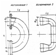
Рис. 3 Калач соединительный
