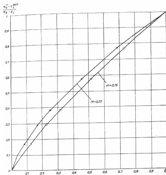
Рис. 3. Графики изменения температурного критерия системы отопления по температуре воды в обратном трубопроводе \left( \frac{\tau_{21}^T - t_i^{\text{OPT}}}{\tau_{21}^T - t_i} \right) при постоянной циркуляции воды в системе
