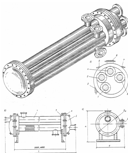
Рис. 5 Общий вид горизонтального многоходового кожухотрубного водоподогревателя
